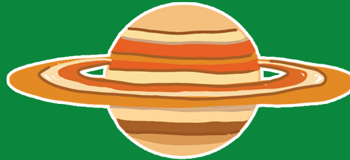
SATURNE (SATURN)
