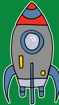
FUSÉE (ROCKET)
